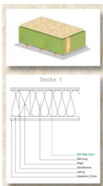
Aufbau oberste Geschossdecke beim Kaldt Dach
